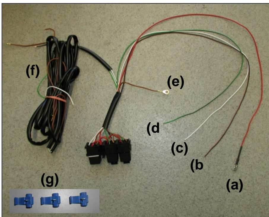
Bild 1: Leitungssatz Frontspoiler mit Abbiegelicht Serie Fig 1: wiring harness front spoiler with turning light as standard
