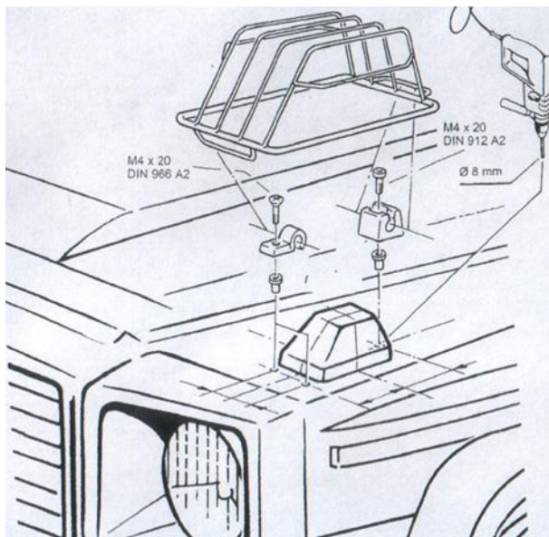
Bild 2: Position der Bohrungen auf Kotflügel Fig. 2: Positions of the drill-holes on the fender
