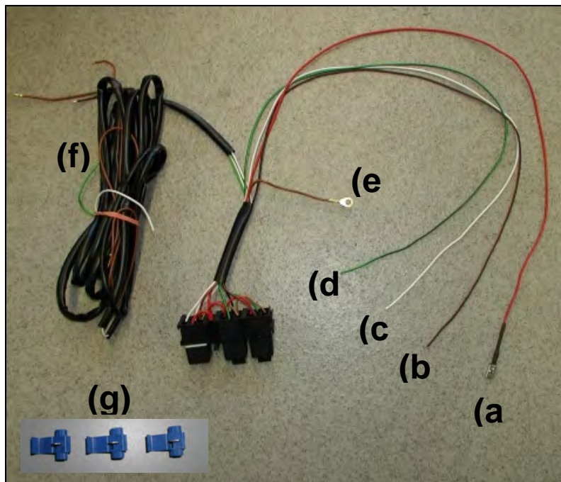
Bild 1: Leitungssatz Frontspoiler mit Abbiegelicht Serie
