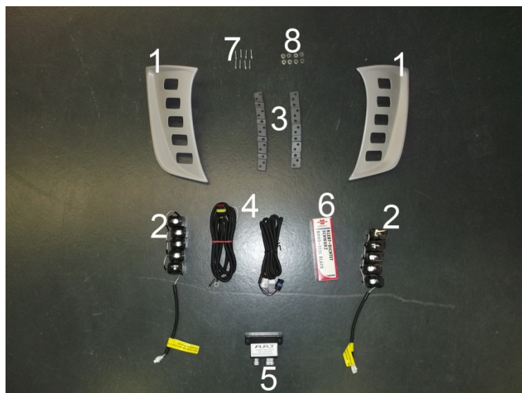
Bild 2: Lieferumfang DL03 463 00 Figure 2: Items supplied DL03 463 00
