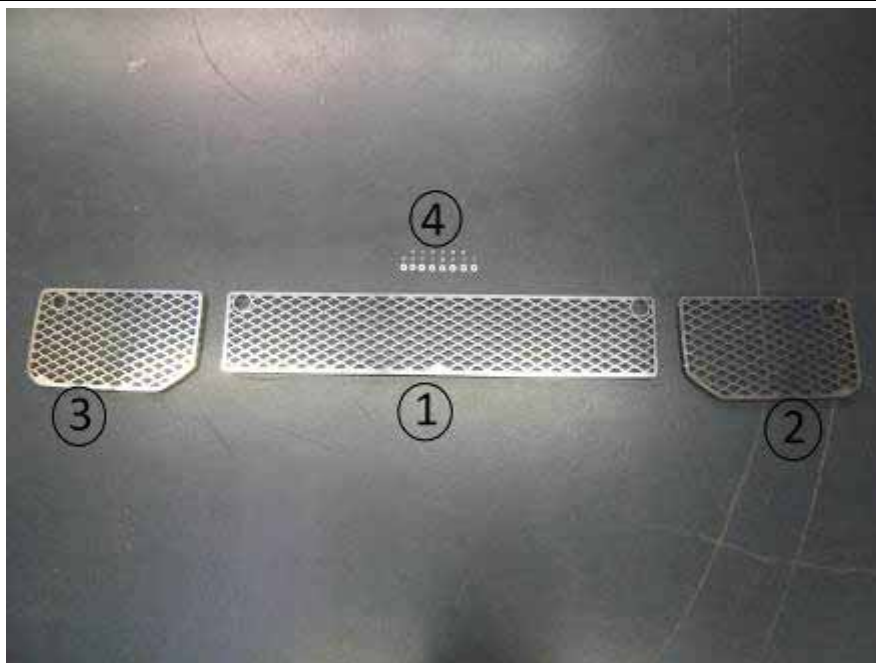
Bild 1: Lieferumfang APEG 463 63 Figure 1: Items supplied APEG 463 63
